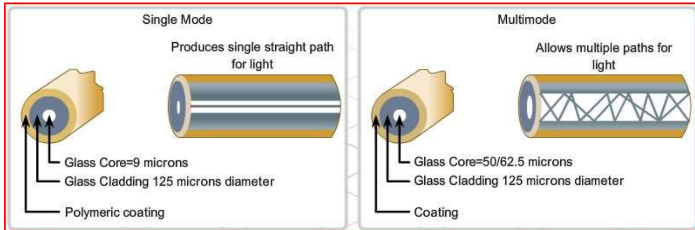
Fig. 2.14 Fire de fibră optică
