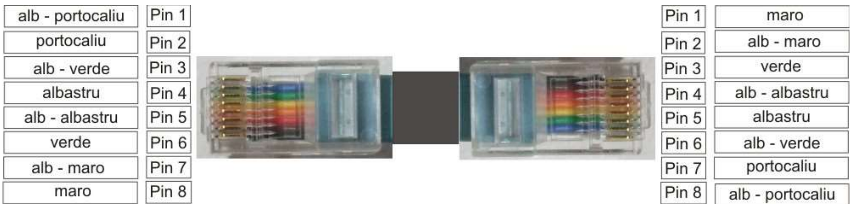
Fig. 8.4 Ordinea firelor într-un cablu Rollover (cablu consolă)
