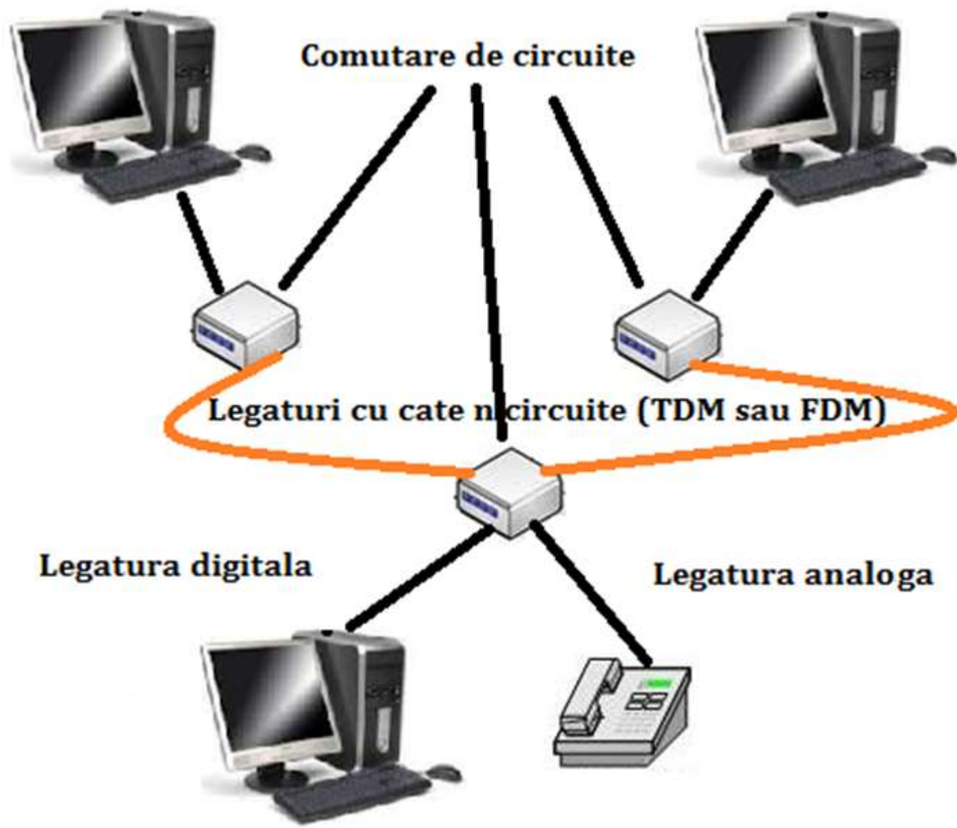
Fig. 4 Rețea bazată pe comutare de circuite Rețele de calculatoare
