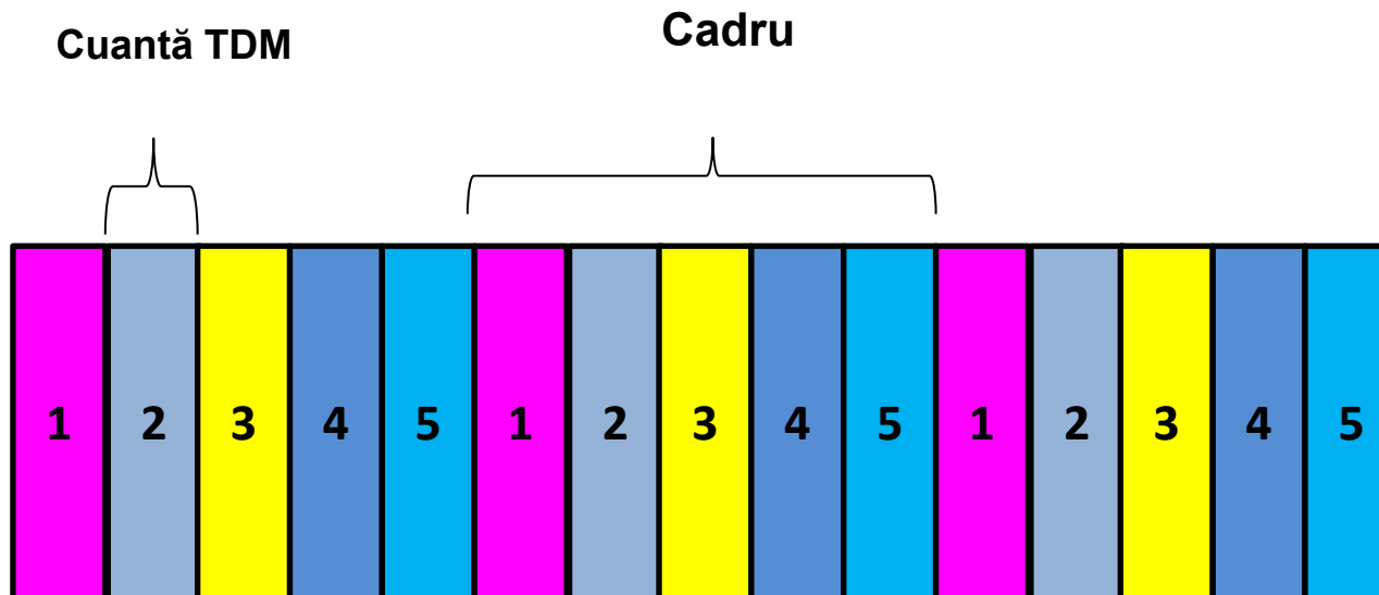
Fig. 6 Multiplexare prin divizarea timpului (TDM)
