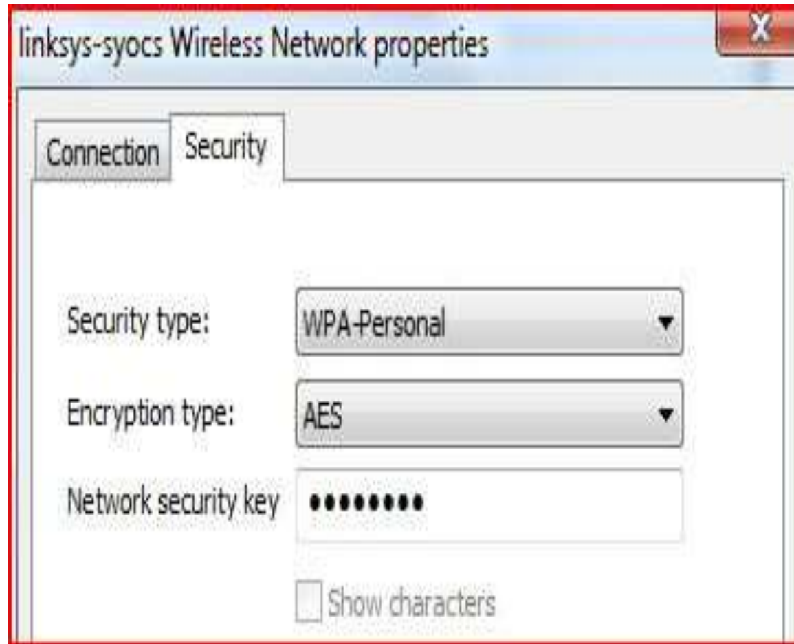
Fig. 7.6 Panou de informații care afișează modul de securitate și tipul criptării a unui
